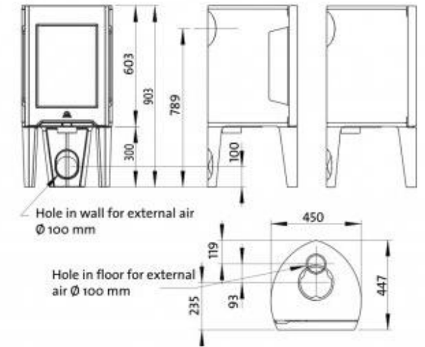
Jøtul F 162 / Jøtul F 163
